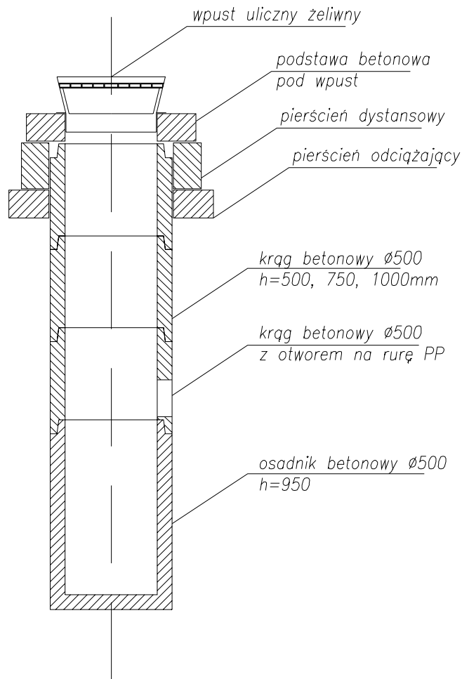
Rysunek poglądowy wpustu ulicznego \varnothing 500 z pierścieniem odcciążającym i wpustem żeliwnym
