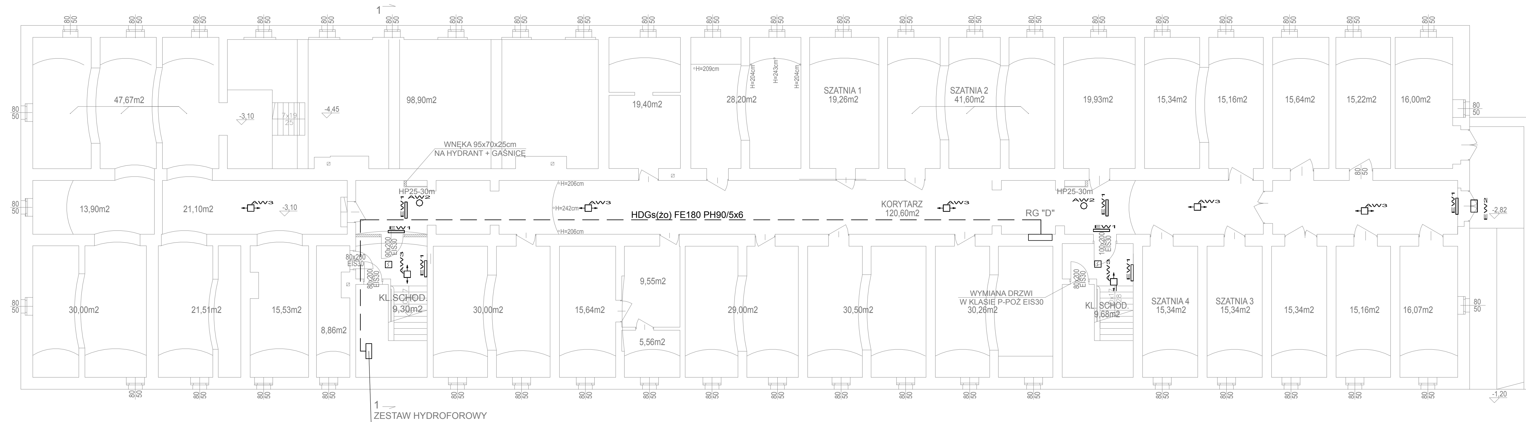
RZUT PIWNIC - STAN PROJEKTOWANY 1:100 BUDYNEK "D"
