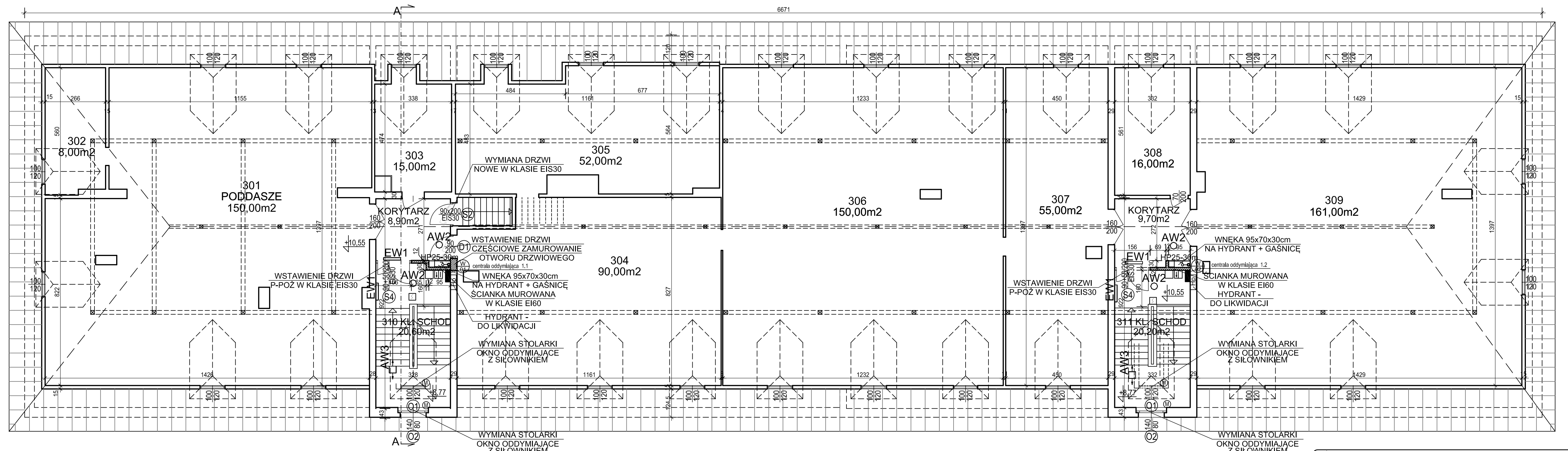
RZUT PODDASZA - STAN PROJEKTOWANY 1:100 BUDYNEK "D"
