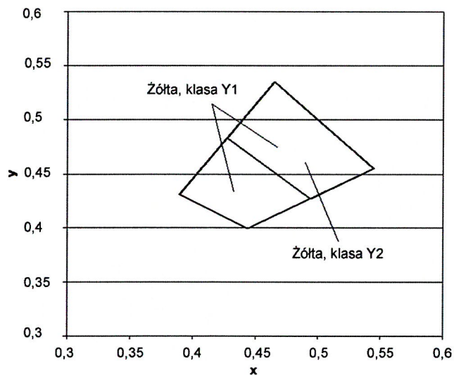
Rys.2. Współrzędne chromatycywności x,y dla barwy żółtej oznakowania
