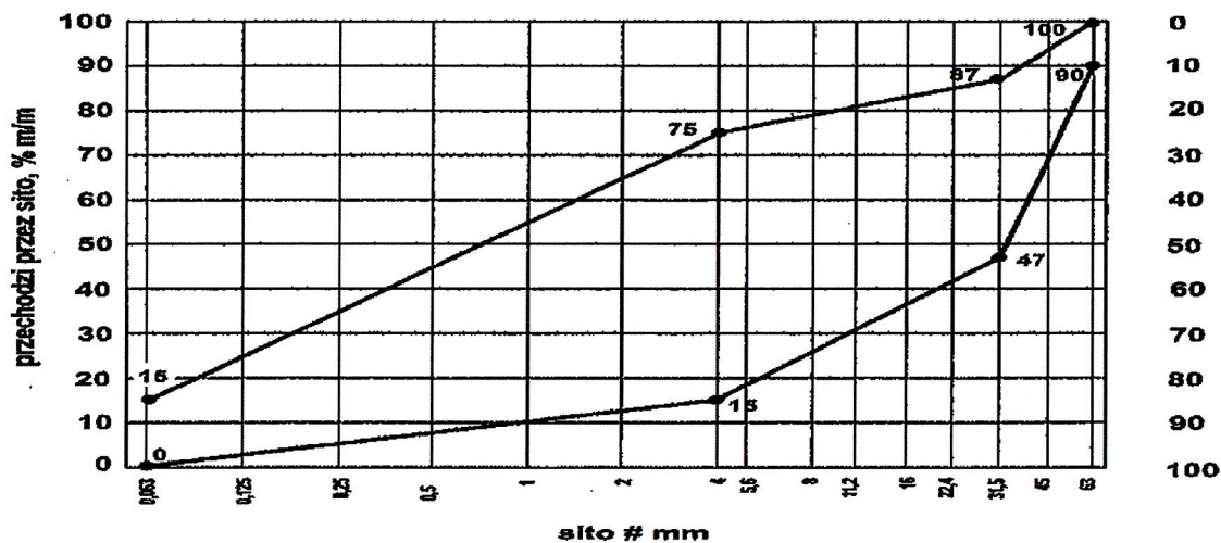
Rys. 8. Mieszanka kruszywa 0/63 do górnej warstwy podłoża ulepszonego /warstwy mrozoochronnej
