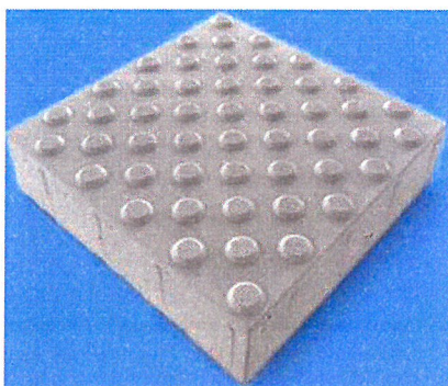
Rys. 2a. Płytką ostrzegawcza (pole decyzji)– szczegół powierzchni
